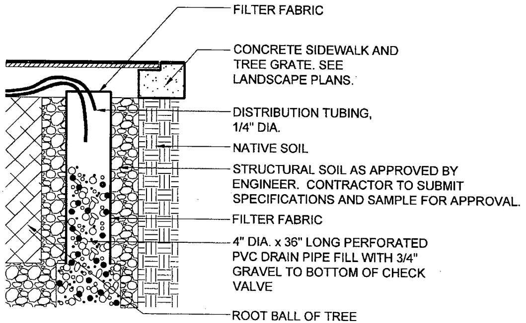
SECTION VIEW - N.T.S.
