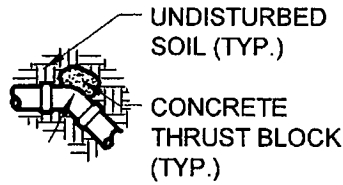
11-1/4°, 22-1/2° OR 45° BENDS
